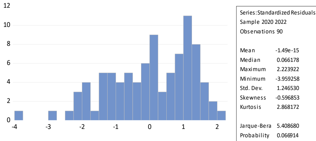
Gambar 2. Uji Normalitas
